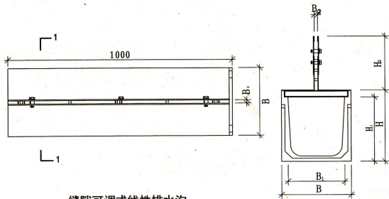
缝隙可调式线性排水沟
