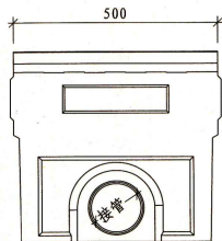
2-2剖面图
