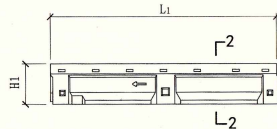
企口U型排水沟沟底仰视图
