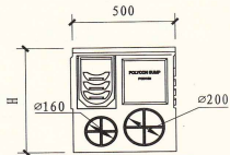
企口集水井立面图
