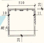
2-2剖视图
