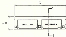
平口U型排水沟立面图
