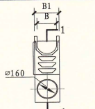
平口集水井侧视图
