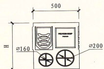
平口集水井立面图
