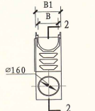
企口集水井侧视图
